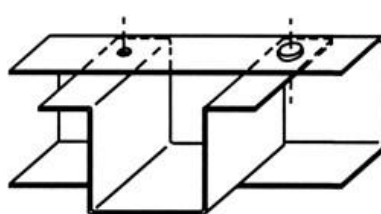
Kloboukový profil v profilu U s přírubovými spoji
