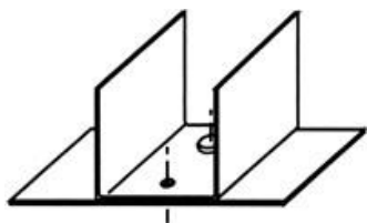
Profil U na plechu se stojinovým spojením
