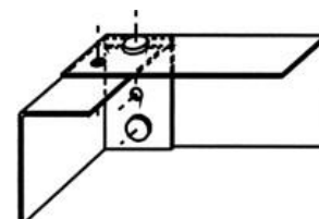
Diagonální rohový spoj s přesahem ramen
