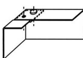
Diagonální rohový spoj s přesahem 2
