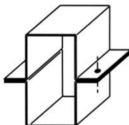
Spoj s dvojitým klobúkovým profilom
