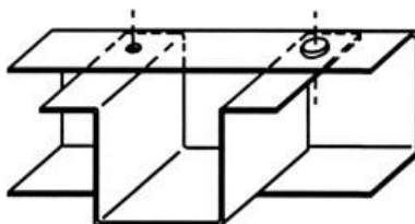
Klobúkový profil v profile U s prírubovými spojmi
