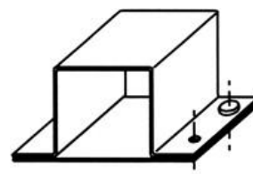
Klobúkový profil na plechu s prírubovými spojmi
