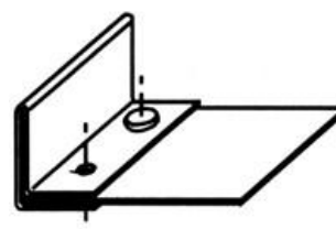
Połączenie narożne diagonalne z zakładką ramion
