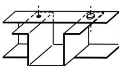
Profil kapeluszowy w profilu U z połączeniami kołnierzowymi
