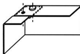
Połączenie narożne diagonalne z zakładką 2
