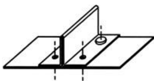
Profil w kształcie T z blachą z połączeniem kołnierзовym
