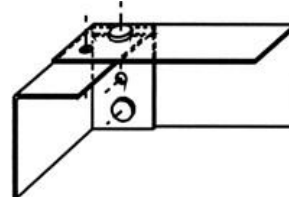
Połączenie narożne diagonalne z zakładką ramion
