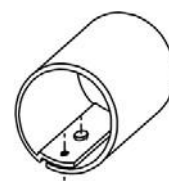
Zakładane połączenie rur okrągłych
