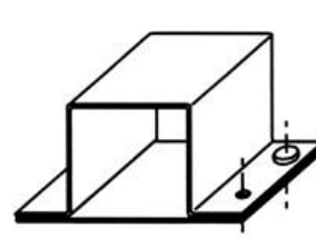
Profil kapeluszowy na blasze z połączeniami kołnierzowymi
