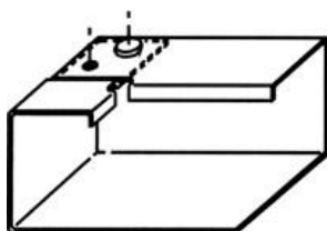
Połączenie narożne diagonalne z wewnętrzną krawędzią
